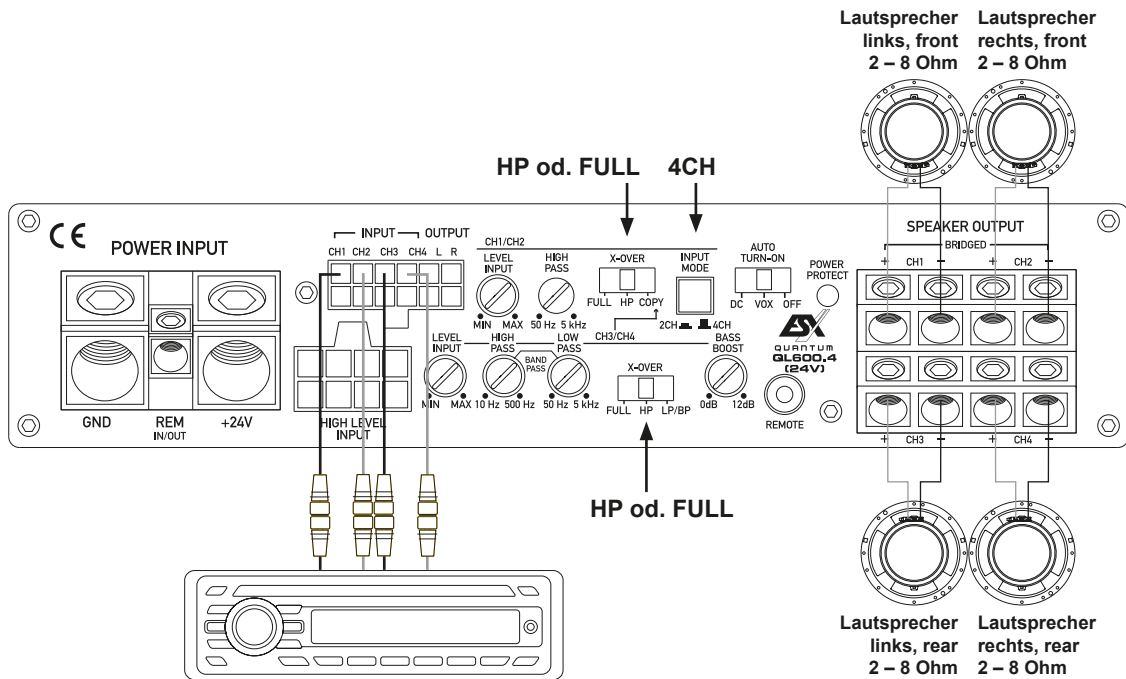
Stereo Cinch-Audiokabel (FL/FR & RL/RR) vom Steuergerät mit INPUT CH1 / CH2 und CH3 / CH4 des Verstärkers verbinden
